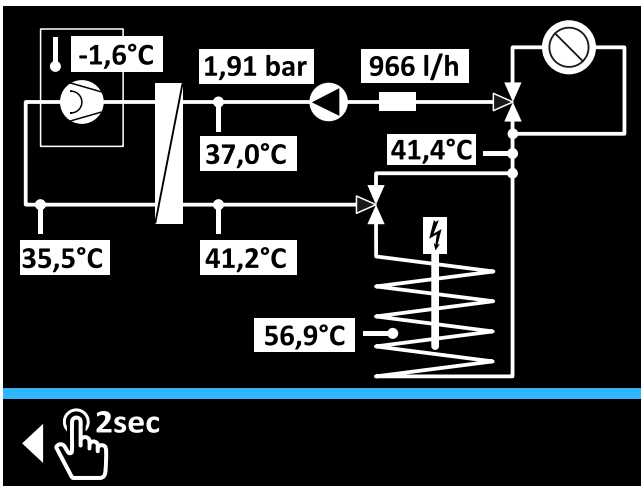
4-8 Hydraulikschaltbild - Zweite Seite
