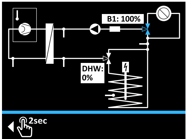
4-9 Hydraulikschaltbild - Dritte Seite
