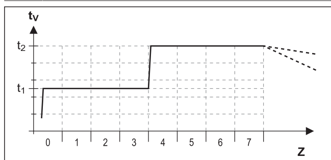
4-5 Zeitlicher Ablauf des Estrichprogramms beim Funktionsheizen
