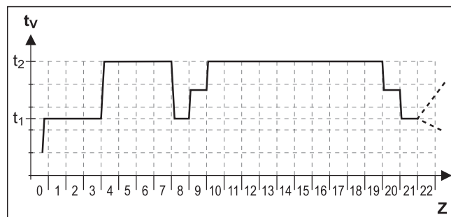
4-6 Zeitlicher Ablauf des Estrichprogramms beim kombinierten Funktions- und Belegreifeheizen
