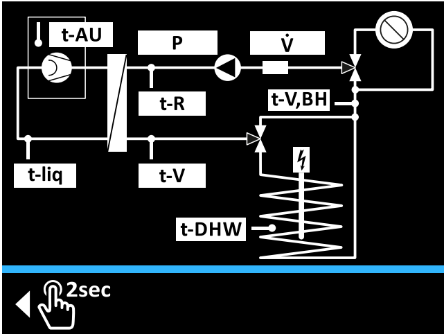
4-7 Hydraulikschaltbild - Erste Seite
