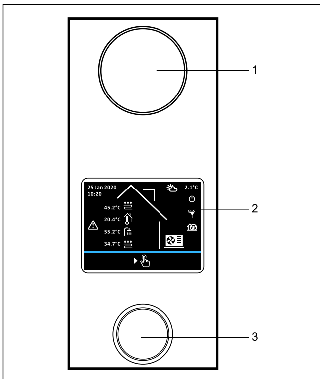
3-1 RoCon+ B1 Anzeige- und Bedienelemente
