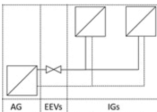
Schema für FDS-Anlagen
