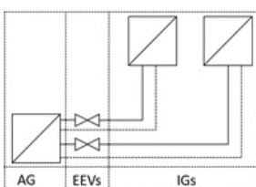
Schema für SX-Anlagen
