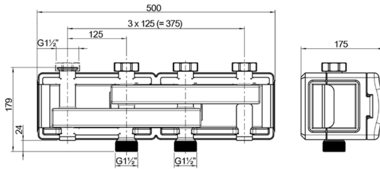
2-fach Verteiler
