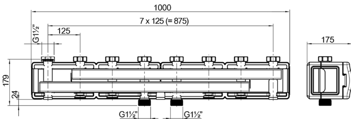
4-fach Verteiler
