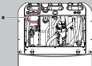
a Kältemittelgasrohr
