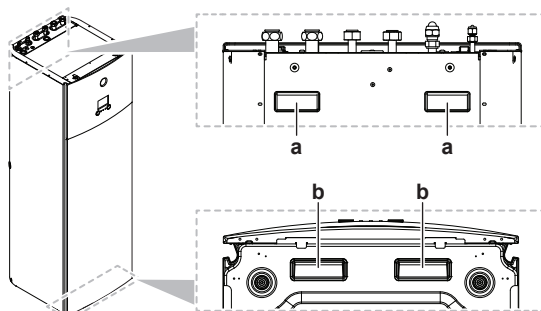
a Griffe an der Rückseite des Geräts
