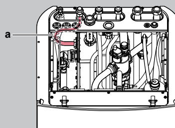
a Kältemittelgasrohr
