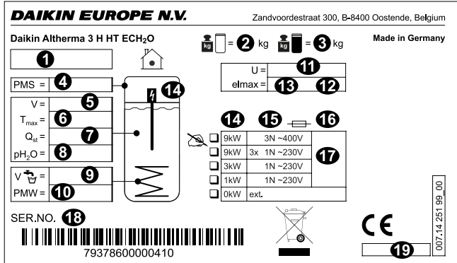
Bild 9-1 Typenschild 1 Geräte-Typ 2 Leergewicht 3 Gesamtgewicht gefüllt 4 Max. zulässiger Betriebsdruck PMS (Heizung) 5 Speicherinhalt gesamt 6 Max. zulässige Betriebstemperatur T_{max}
