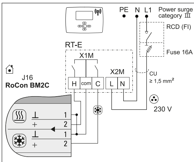
Bild 3-43 Anschluss mit Funk-Raumthermostat (RT-E = Daikin EKRTTR)
