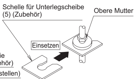
Fixierverfahren für Unterlegscheibe Abb. 16
