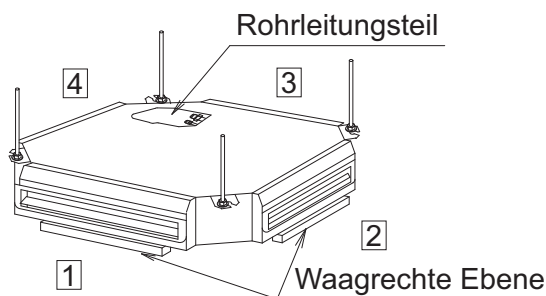
Waagrechte Lage muss sichergestellt sein Abb. 18
