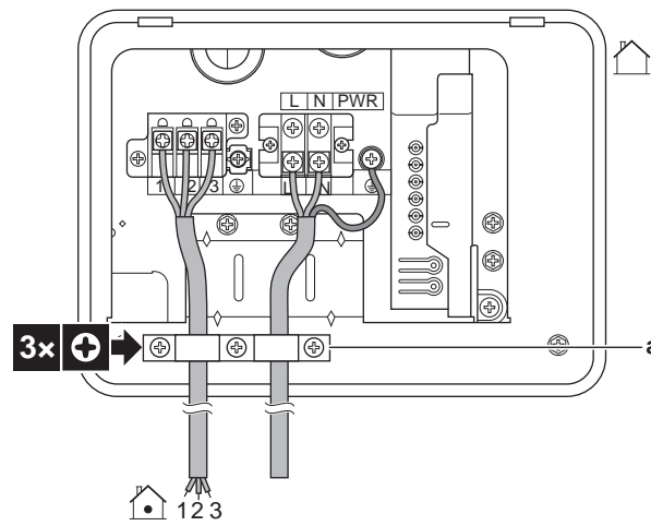
a Drahtklemme
