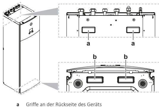
a Griffe an der Rückseite des Geräts
