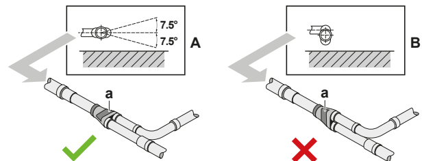
a Warnhinweis Aufkleber ✗ NICHT zulässig ✔ Zulässig
