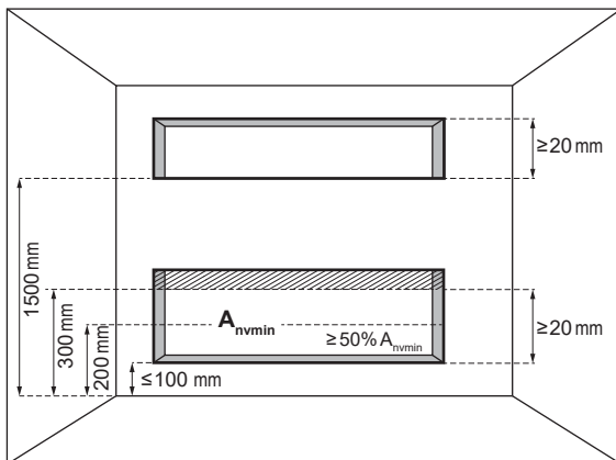
A_{\min} Natürliche Mindestbelüftungsfläche
