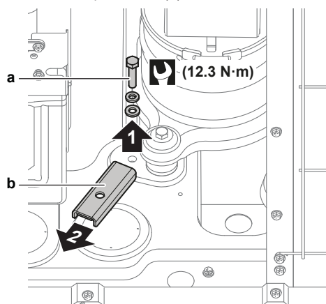
a Bolzen b Transportstütze
