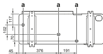
a Kondensatabflusslöcher
