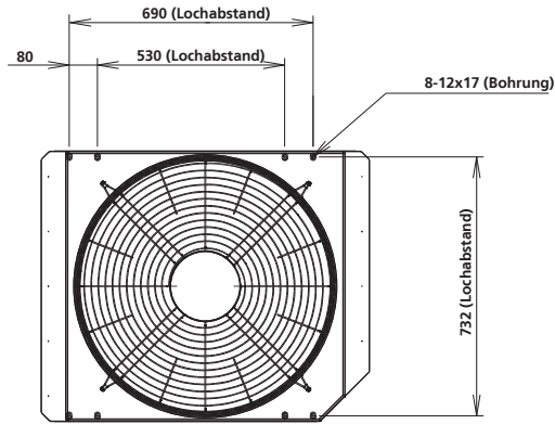
Draufsicht
