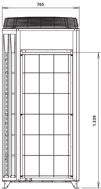
Seitenansicht rechts
