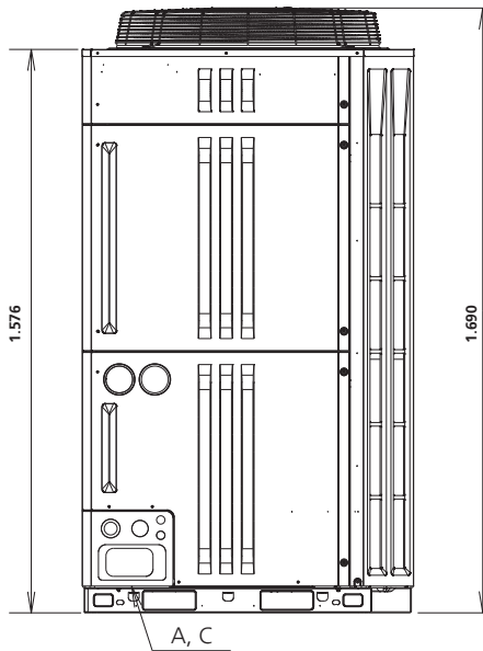
Vorderansicht
