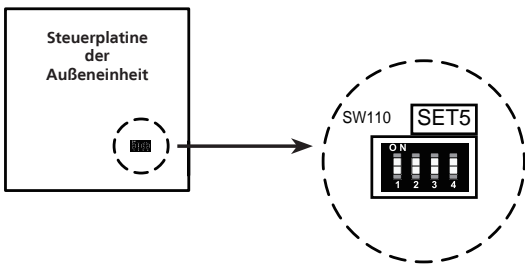
Einstellung Endabschlusswiderstand
