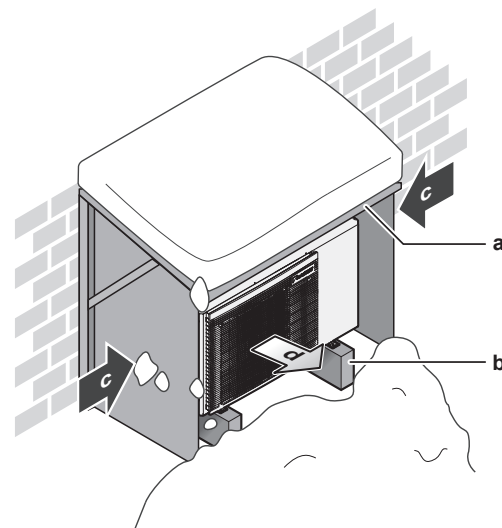
a Schneeabdeckung oder Unterstand b Untergestell c Vorherrschende Windrichtung d Luftauslass
