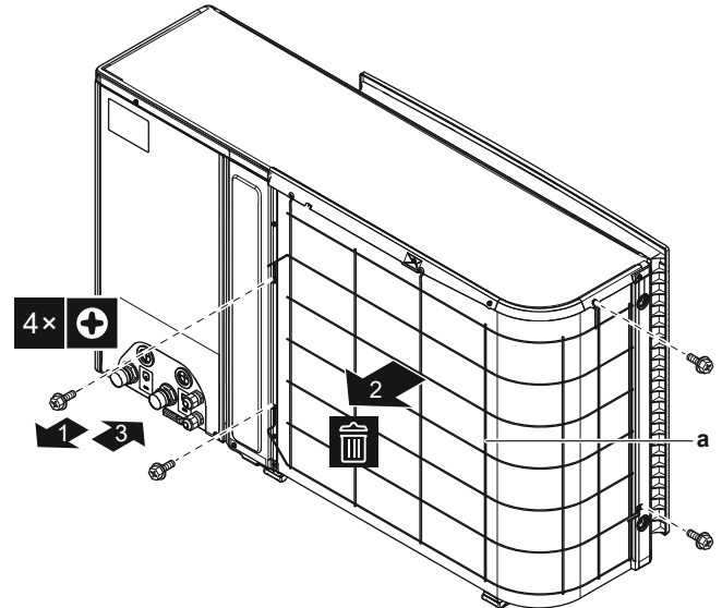
a Ansaugluftgitter
