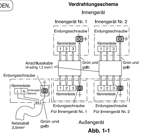
Im Gebäude befindlicher Erdungskabelanschluss zum Außengerät
