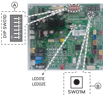
Diagramm Außengeräteplatine
