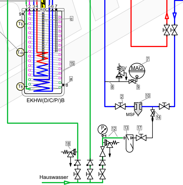
Hygien-Warmwasserspeicher Daikin EKHW
