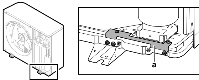
a Transportsicherung
