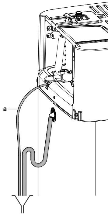
a Ablaufwannenschlauch
