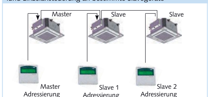
Ansteuerung im Netzwerk mit fünfstufigem Ventilatorbetrieb und Einzelansteuerung an bestimmte Slavegeräte
