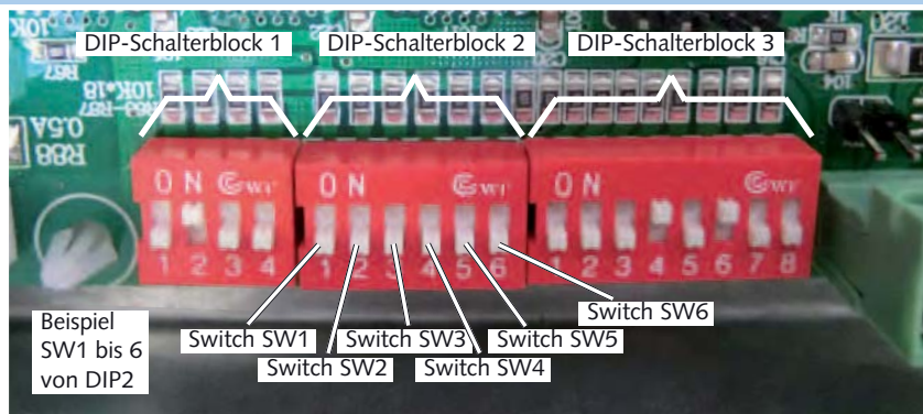
DIP-Schalterblöcke 1 bis 3
