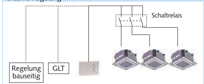
Bedienung mit externem 0...5/10V Signal und stufenlosem Ventilatorbetrieb durch externe Regelung
