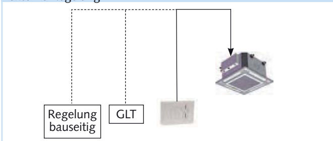
Einzelbedienung mit fünfstufigem Ventilatorbetrieb über IR- oder alternative Kabel-Fernbedienung
