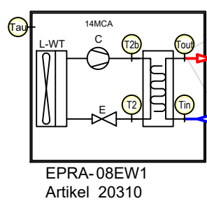
Daikin Altherma 3 R H MT W Artikel 20986 (20310+20958)
