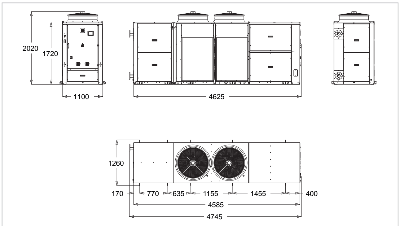
Abb. 9: Abmessungen KWE 1150-1550 mit Speicher (Alle Angaben in mm)
