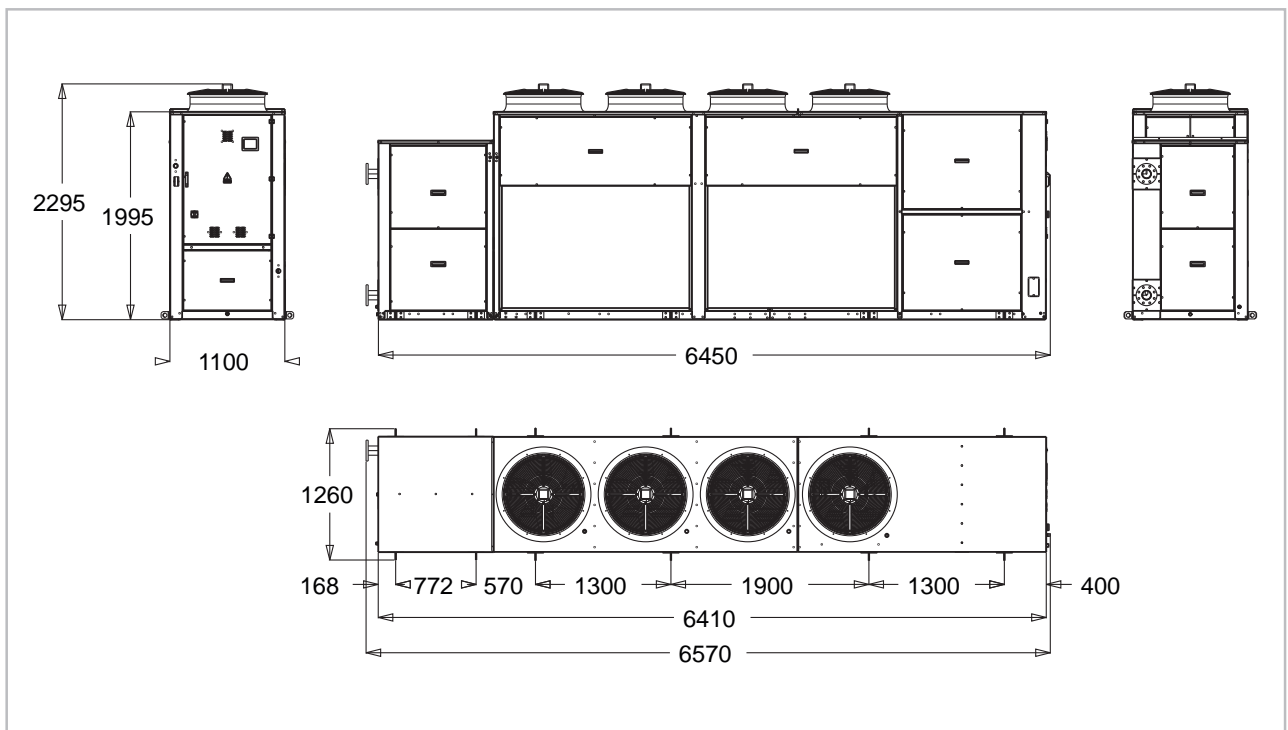
Abb. 13: Abmessungen KWE 2600-3150 mit Speicher (Alle Angaben in mm)
