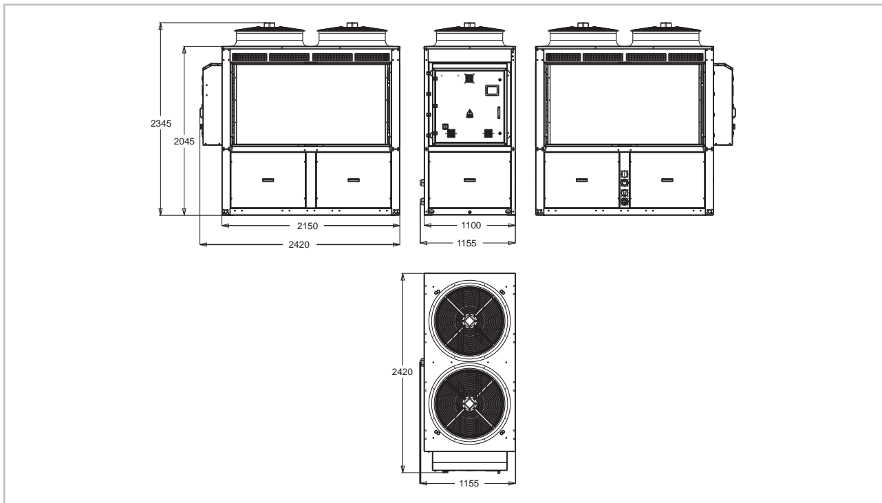
Abb. 6: Abmessungen KWE 970-1060 ohne Speicher (Alle Angaben in mm)
