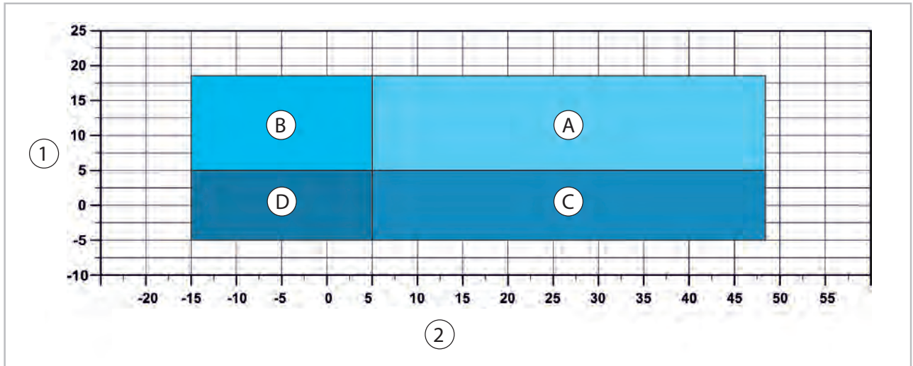
Abb. 1: Einsatzgrenzen
