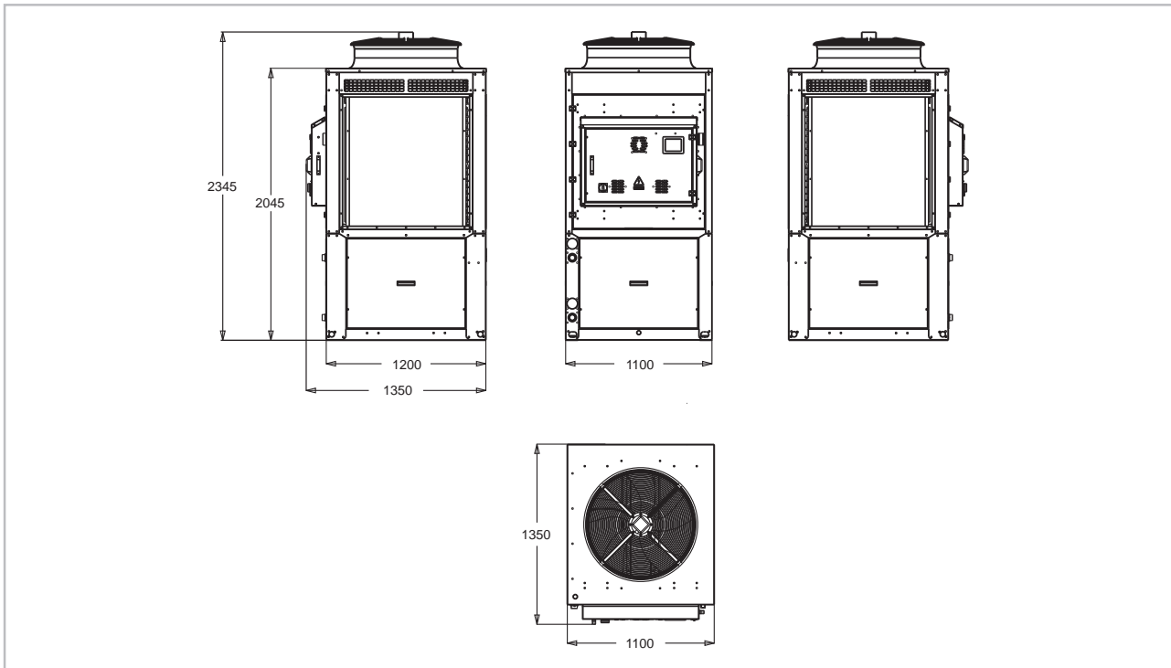
Abb. 2: Abmessungen KWE 290-640 ohne Speicher (Alle Angaben in mm)
