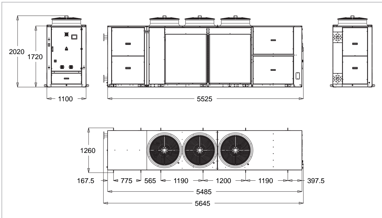
Abb. 11: Abmessungen KWE 1600-2350 mit Speicher (Alle Angaben in mm)
