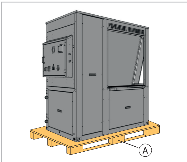
A: Transportpalette
