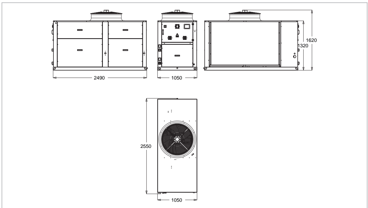
Abb. 5: Abmessungen KWE 730-800 mit Speicher (Alle Angaben in mm)
