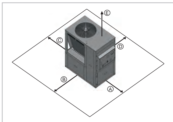
Abb. 16: Mindestfreiräume
