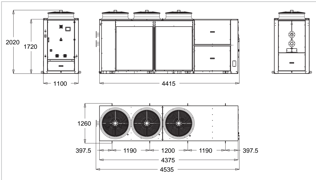
Abb. 10: Abmessungen KWE 1600-2350 ohne Speicher (Alle Angaben in mm)
