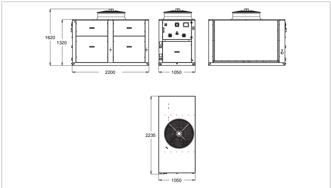
Abb. 4: Abmessungen KWE 730-800 ohne Speicher (Alle Angaben in mm)
