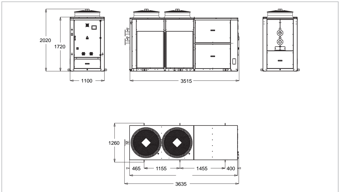
Abb. 8: Abmessungen KWE 1150-1550 ohne Speicher (Alle Angaben in mm)
