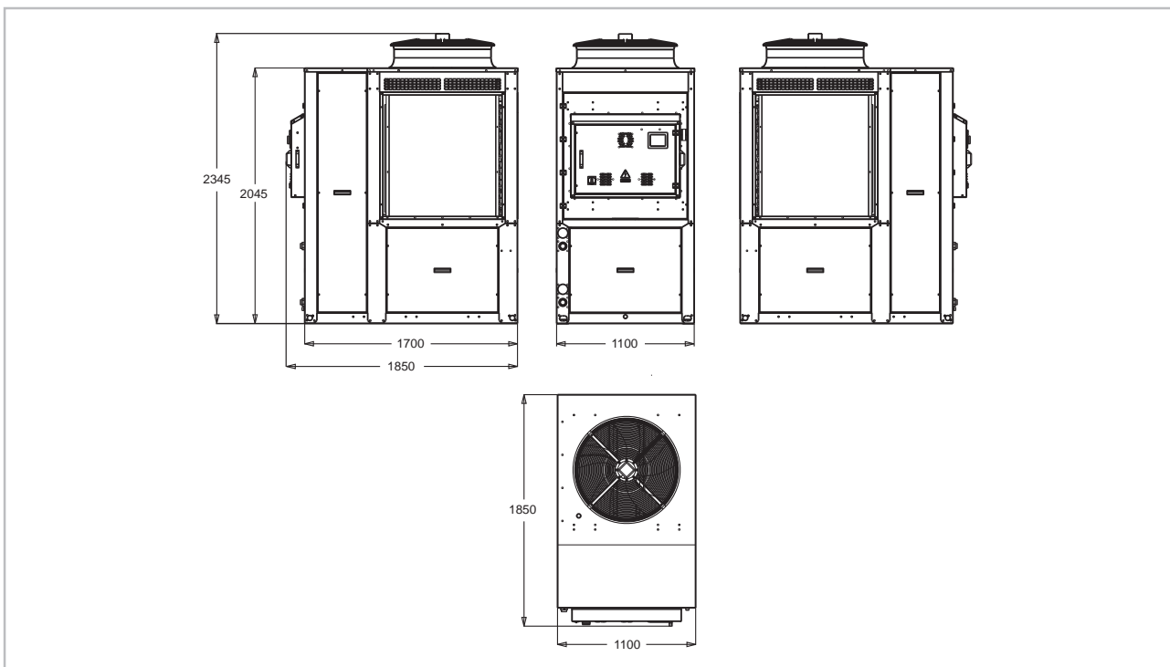
Abb. 3: Abmessungen KWE 290-640 mit Speicher (Alle Angaben in mm)
