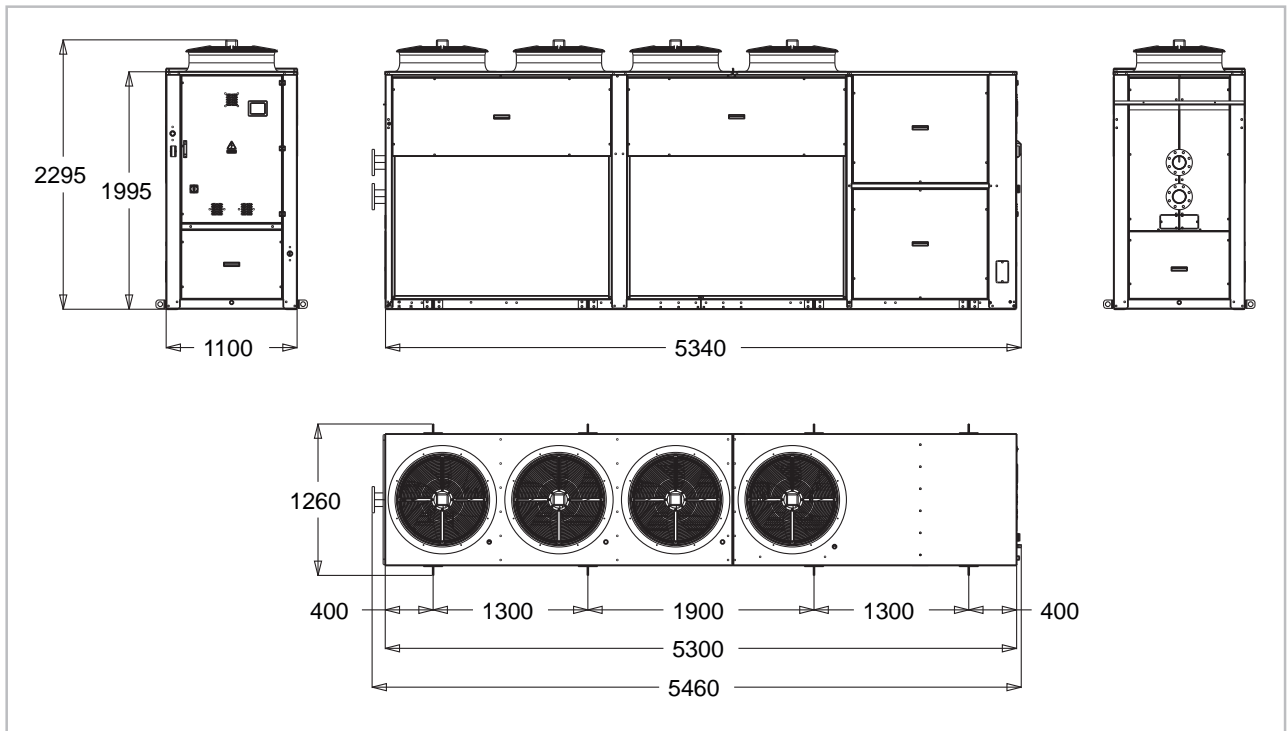
Abb. 12: Abmessungen KWE 2600-3150 ohne Speicher (Alle Angaben in mm)
