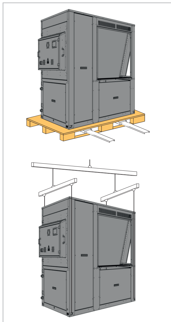
Abb. 15: Gerätetransport
