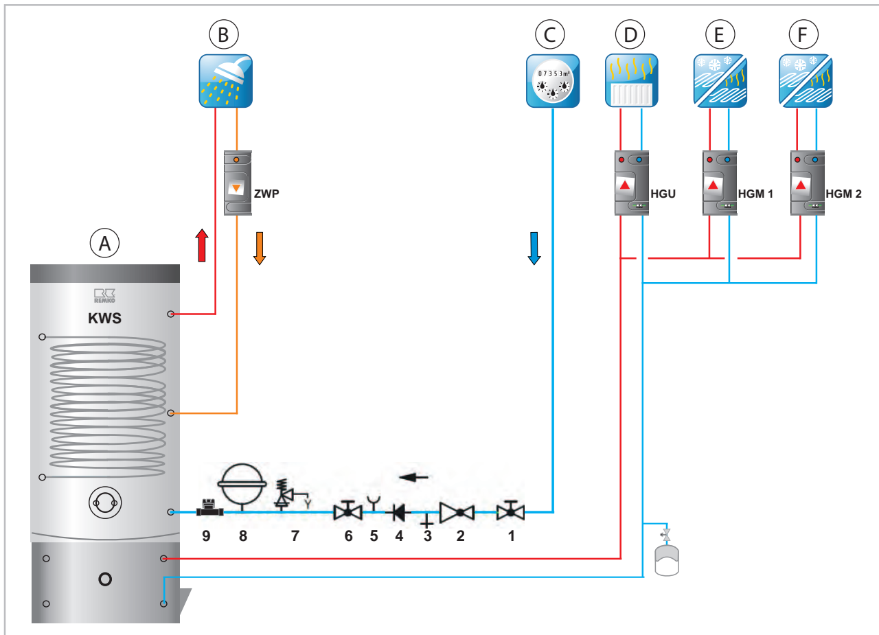
Abb. 4: Speicheranschluss nach DIN 1988
