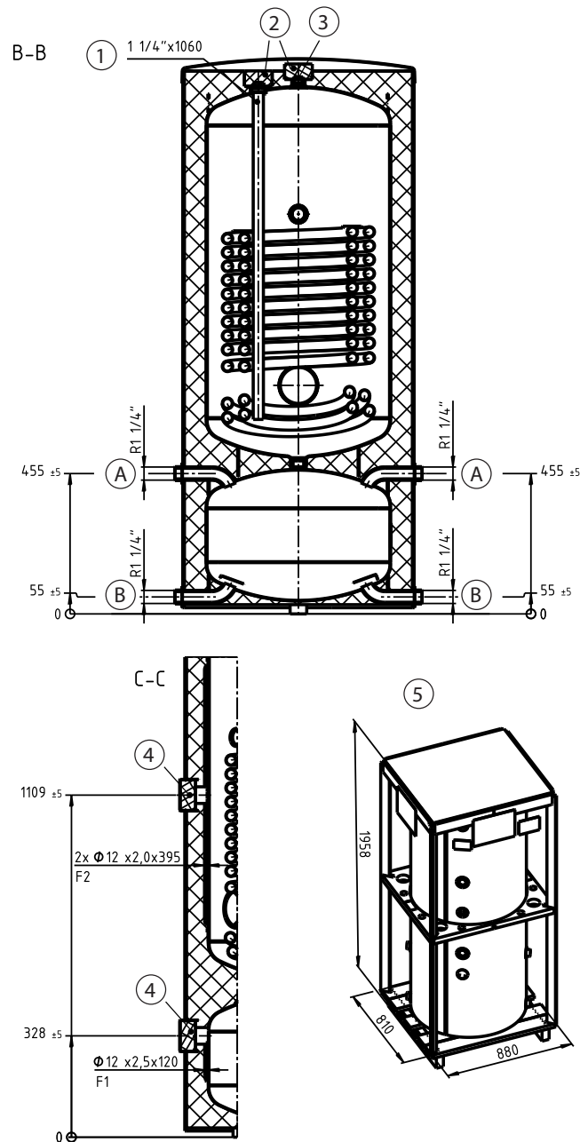
Abb. 2: Geräteabmessungen (Alle Angaben in mm)
