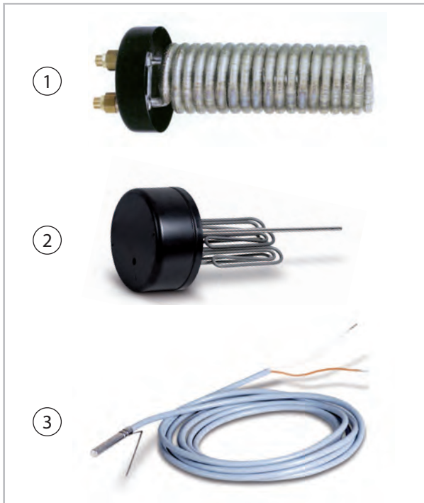
Abb. 6: Ersatzteile
