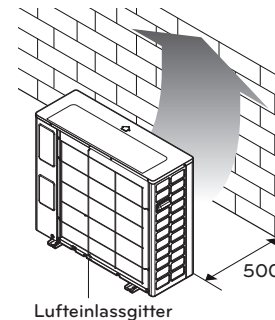
Lufteinlassgitter
