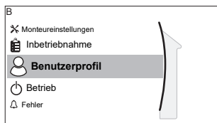
[B] Benutzerprofil
