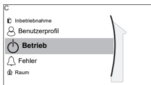
[C] Betrieb
