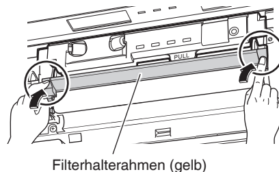
Filterhalterahmen (gelb)
