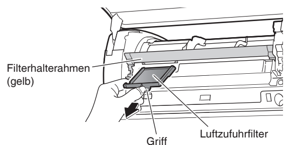
Griff
