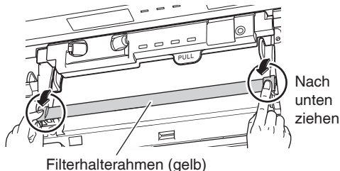
Filterhalterahmen (gelb)
