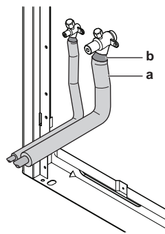
a Isoliermaterial b Abdichten usw.
