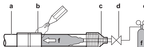
a Kältemittelrohre b Zu verlötendes Teil
