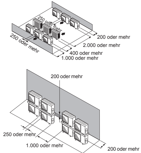
(2) Mehrfach-Parallelgeräteanordnung
