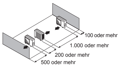
(1) Einzel-Parallelgeräteanordnung
